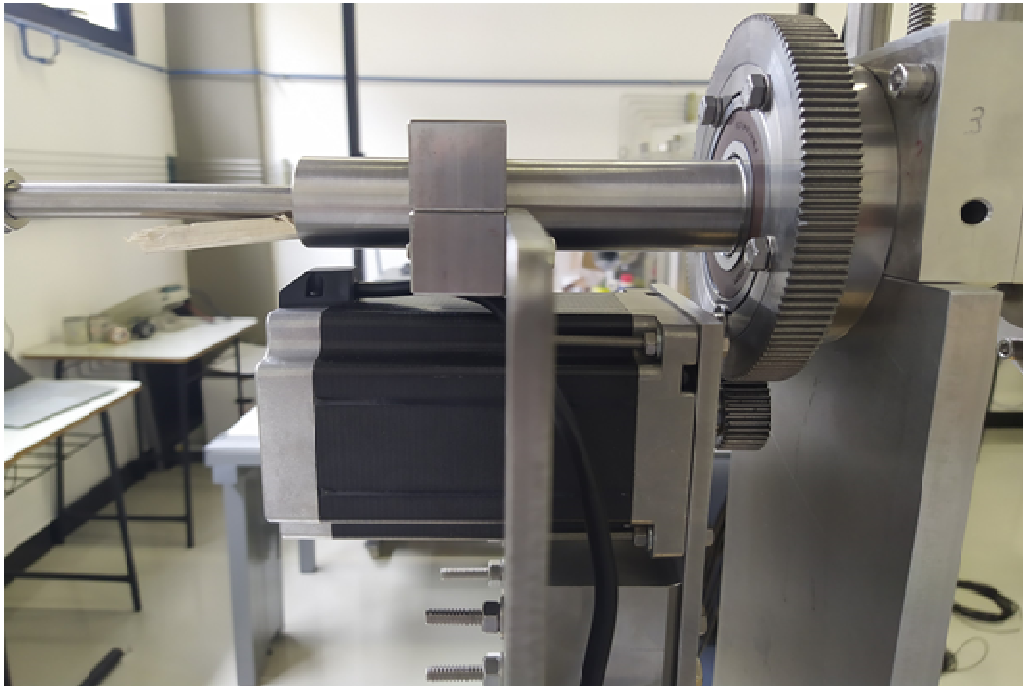
Projeto Petrobras – ESTANQUEIDADE - Detalhe do sistema de movimentação do detector de Hélio – Coordenação Prof. Dr. Argemiro Soares S. Sobrinho
